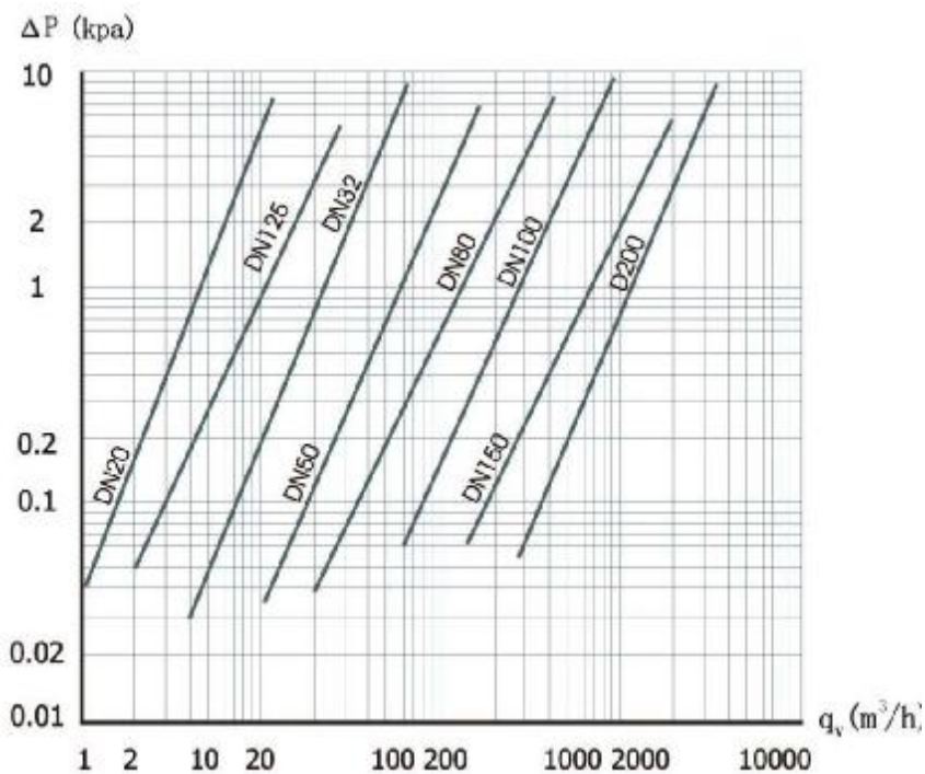
压力损失曲线
