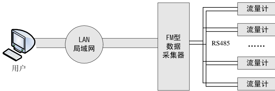
局域网传输
