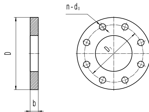
连接法兰
