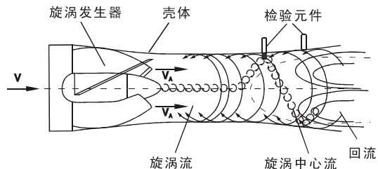
工作原理图
